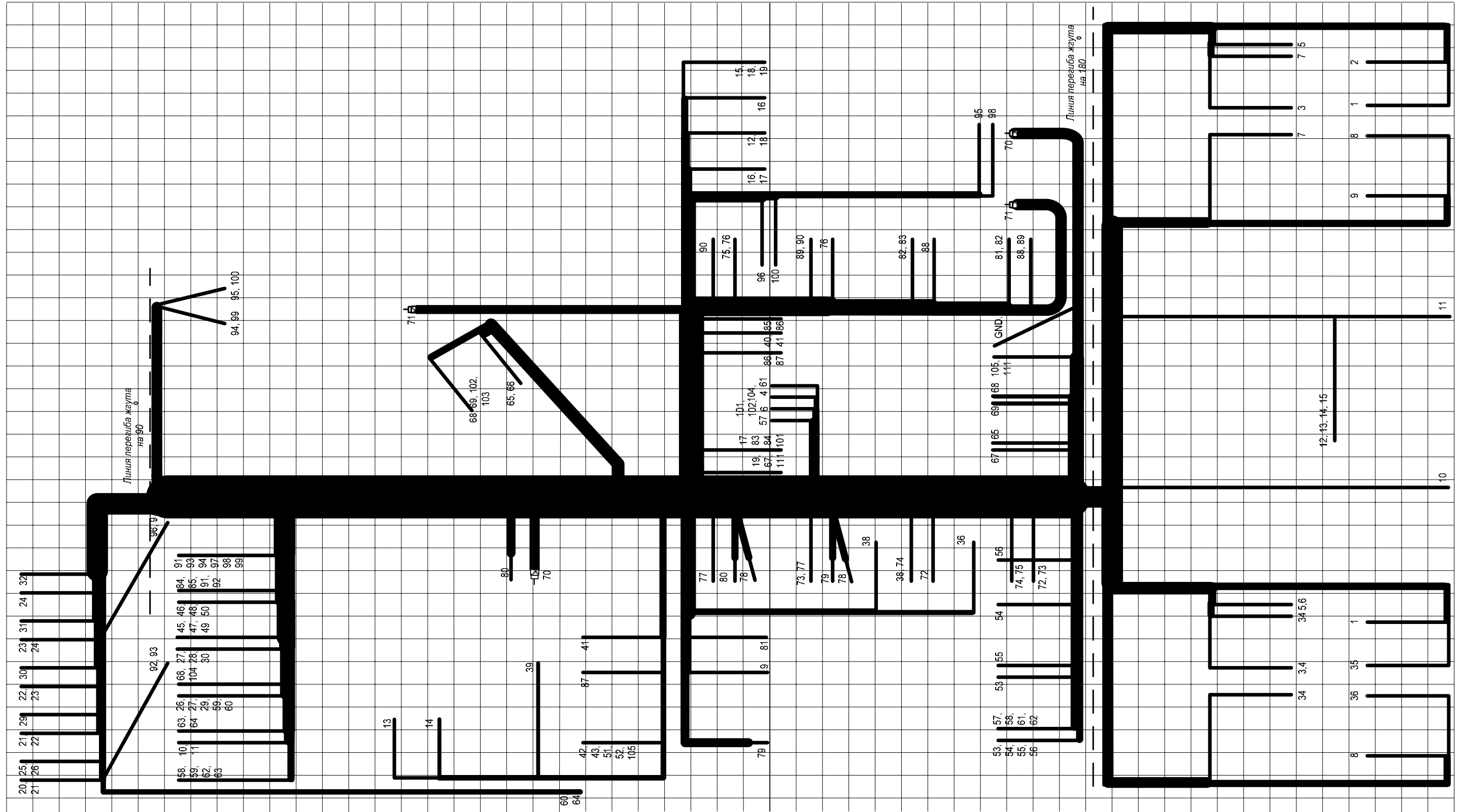
Рис. 14А. Чертёж жгута усилителя мощности на 2-х лампах ГИ-7Б.
